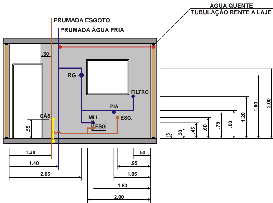
ÁGUA QUENTE TUBULAÇÃO RENTE A LAJE
